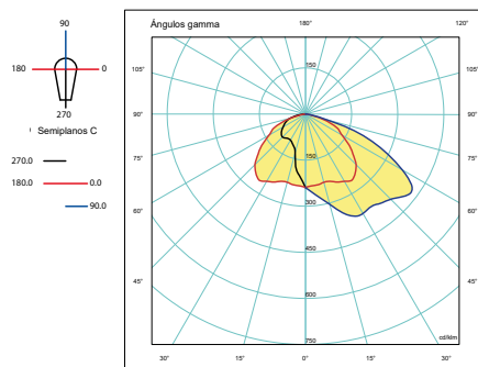
ASY27 CIRKO
