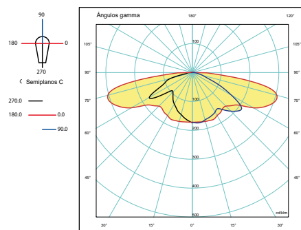
ASY17 CIRKO
