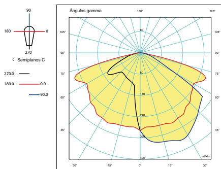
ASY11 CIRKO
