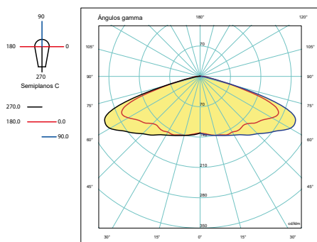
CIR06 CIRKO
