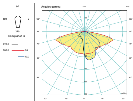
ASY26 CIRKO
