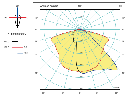
ASY12 CIRKO
